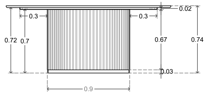
ALZADO A
