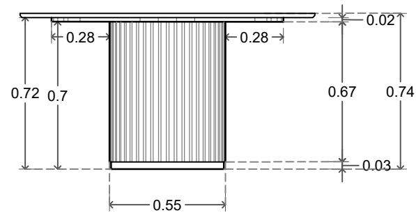
ALZADO A
